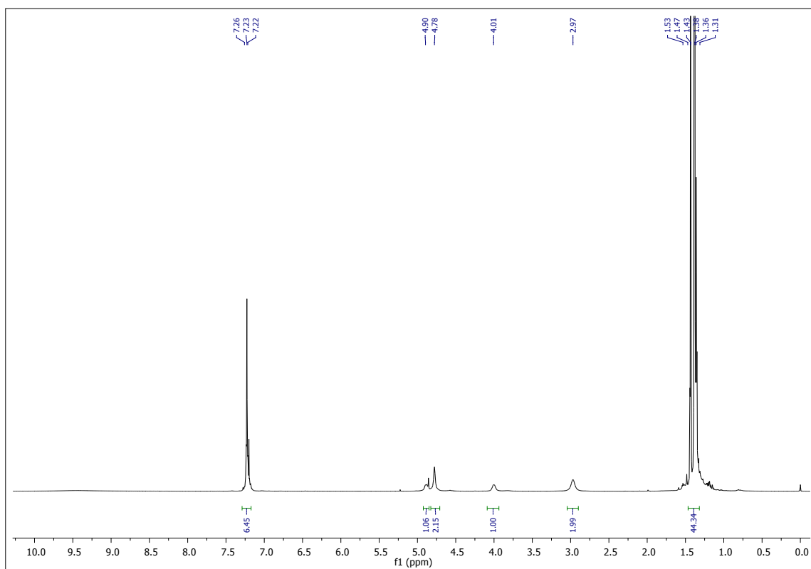
13 C NMR Compound 5e
