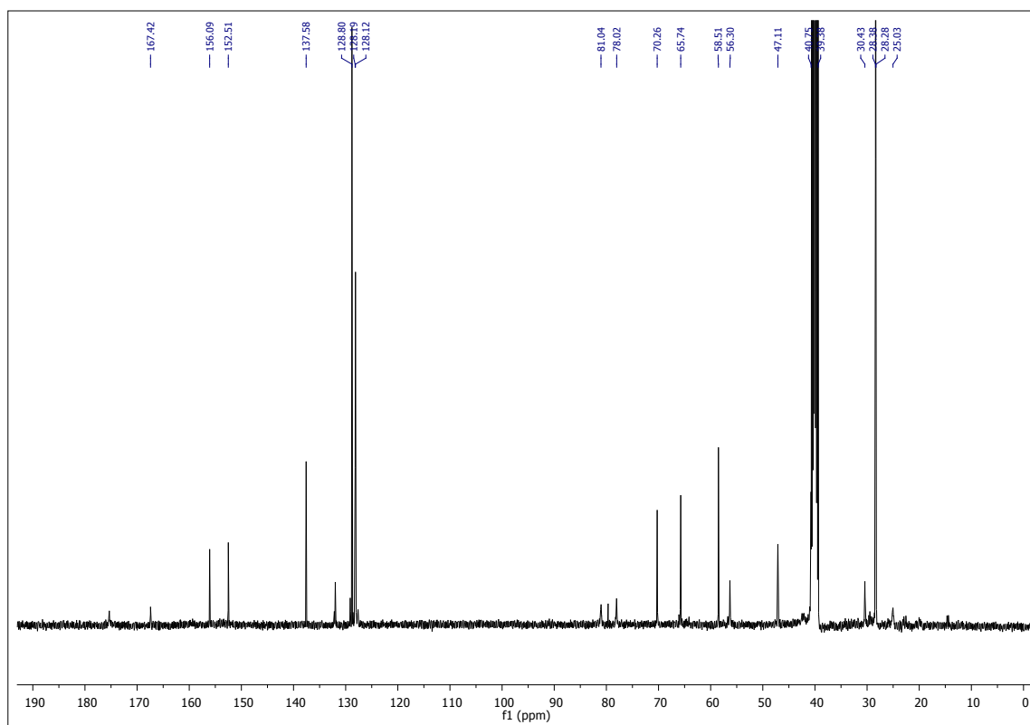
13 C NMR Compound 9a
