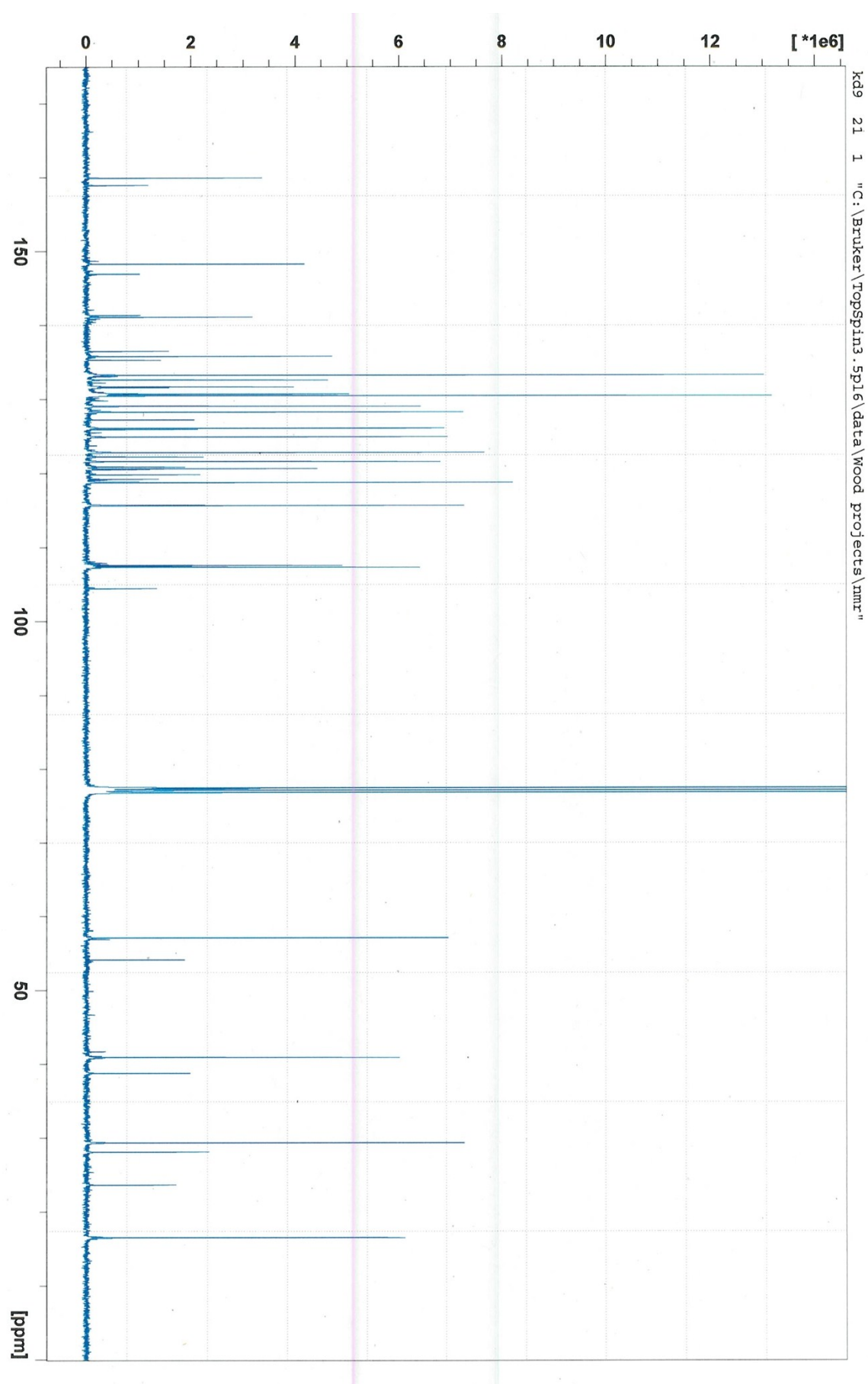
^{13}\text{C} NMR spectrum for 6e
