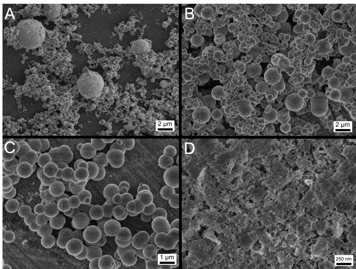
Fig. S1 SEM micrographs of the BiF3 (A), BiF4 (B), BiF5 (C), and BiF8 (D) samples.
