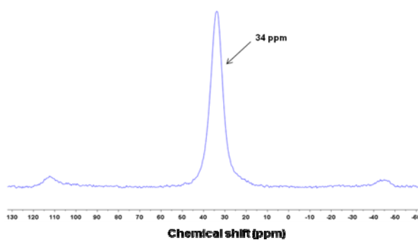
^{31}\text{P} CP-MAS NMR spectrum of M-PO(OEt) 2 10 .
