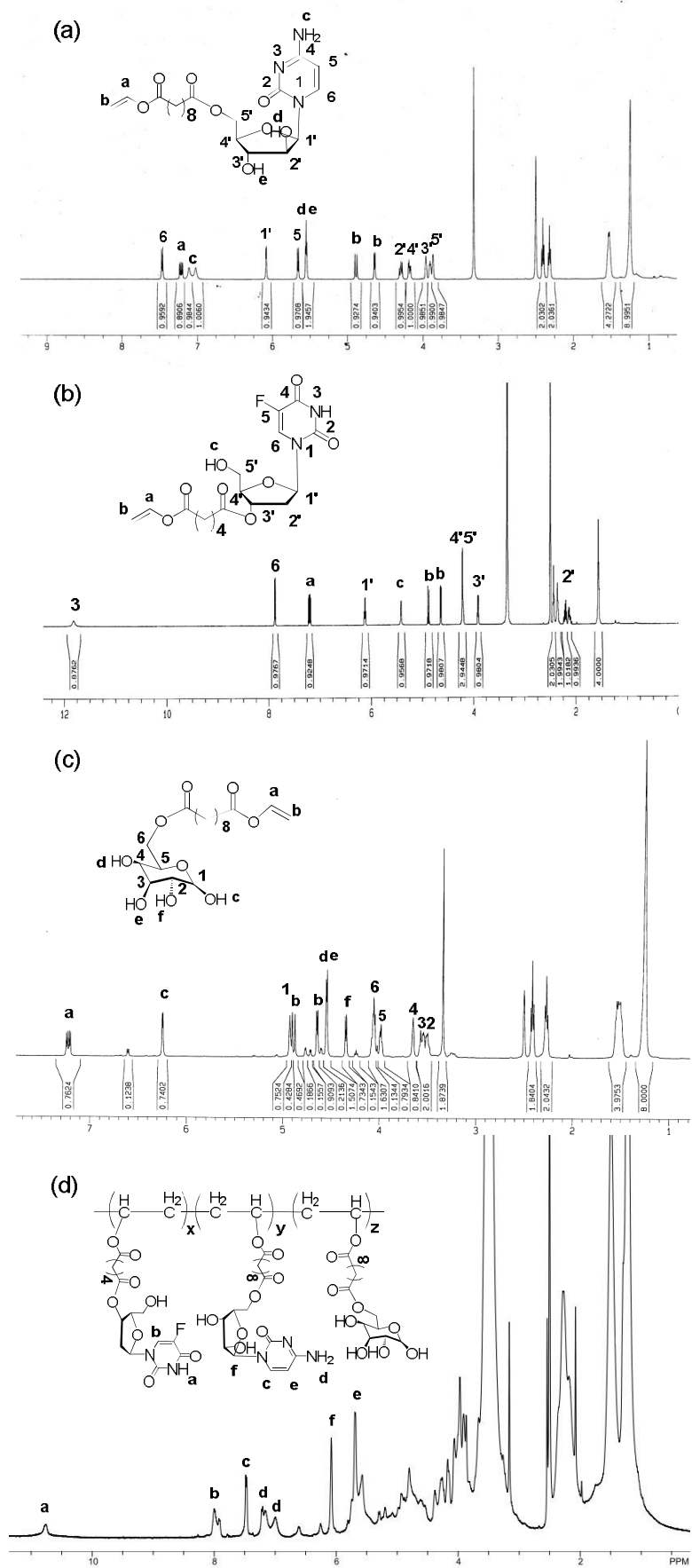
Fig. S2 1 H NMR spectra of (a) VSC, (b) VAF, (c) VGA and (d) poly (VAF-co-VSC-co-VGA).
