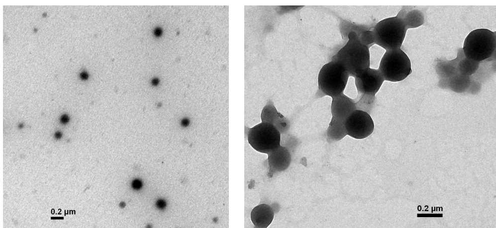
CSO-SA micelles
