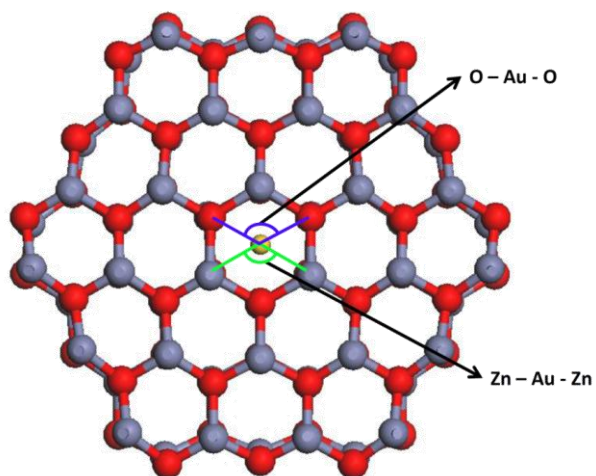
Au Interstitial
