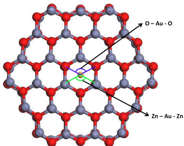
Au Interstitial
