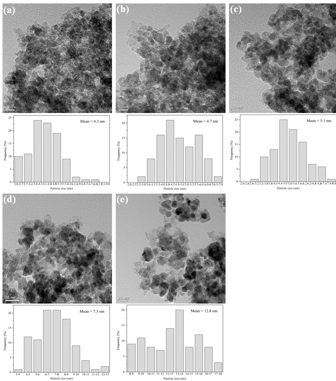
Fig. S1 TEM images of (a) Pd/CZA600, (b) Pd/CZA700, (c) Pd/CZA800, (d) Pd/CZA900, (e) Pd/CZA1000 and the corresponding particle size distributions.
