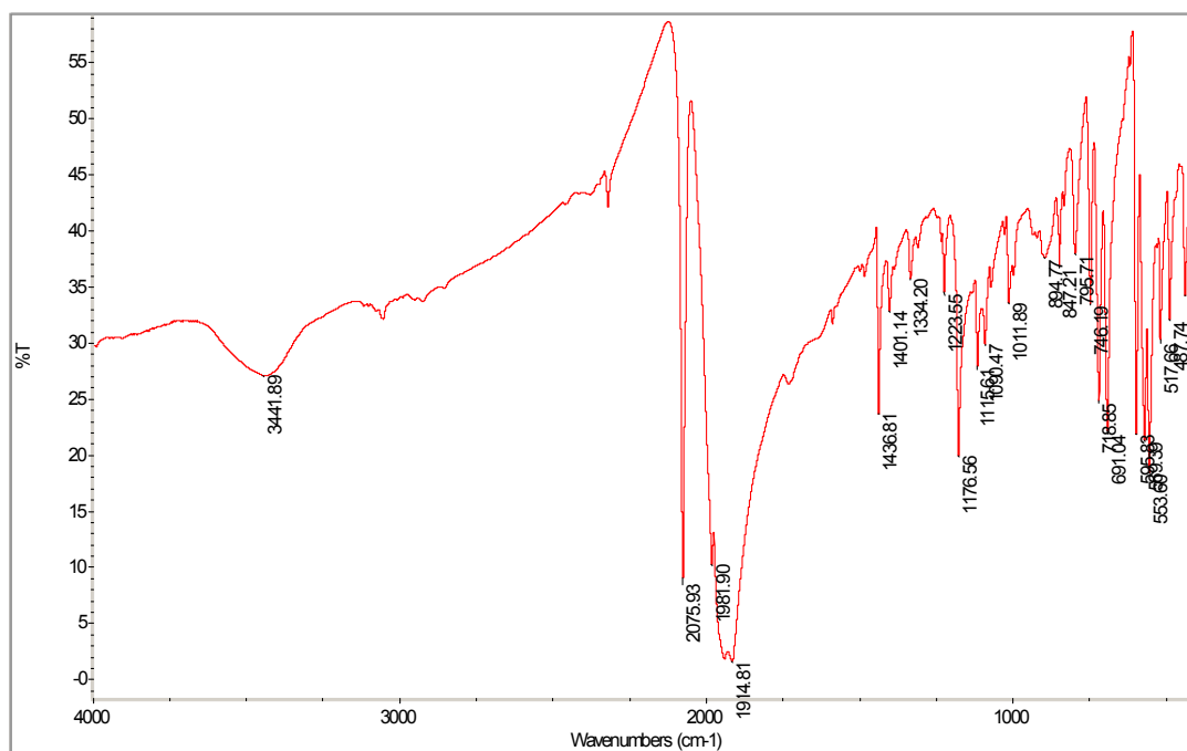
Compound 2e
