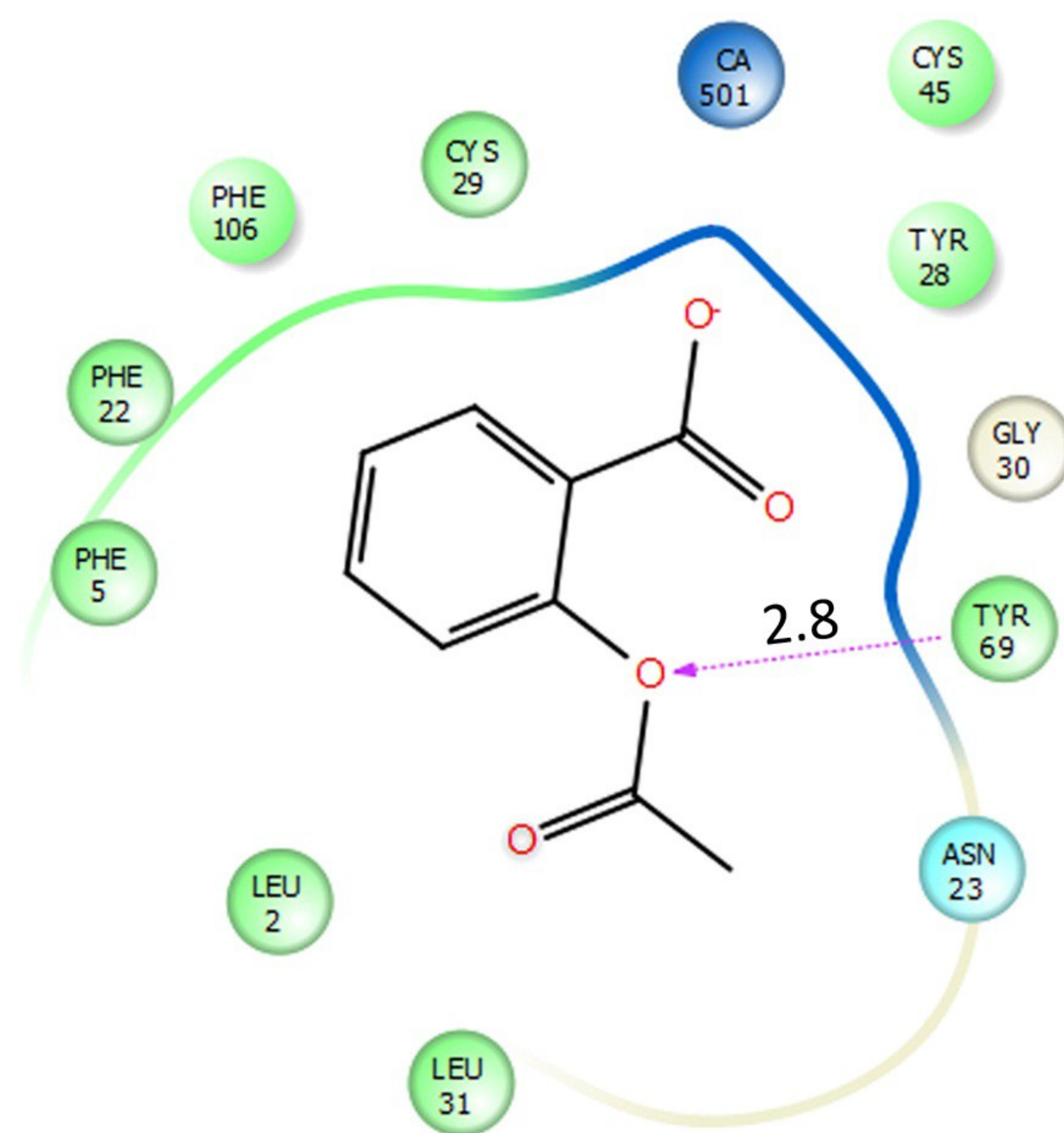
Aspirin
