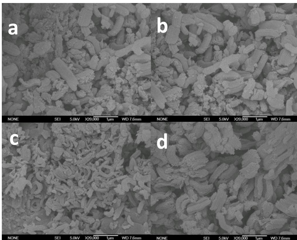
Fig. S2 SEM images of (a) NMC (b) NMC-0.2 (c) NMC-0.5 and (d) NMC-0.8.
