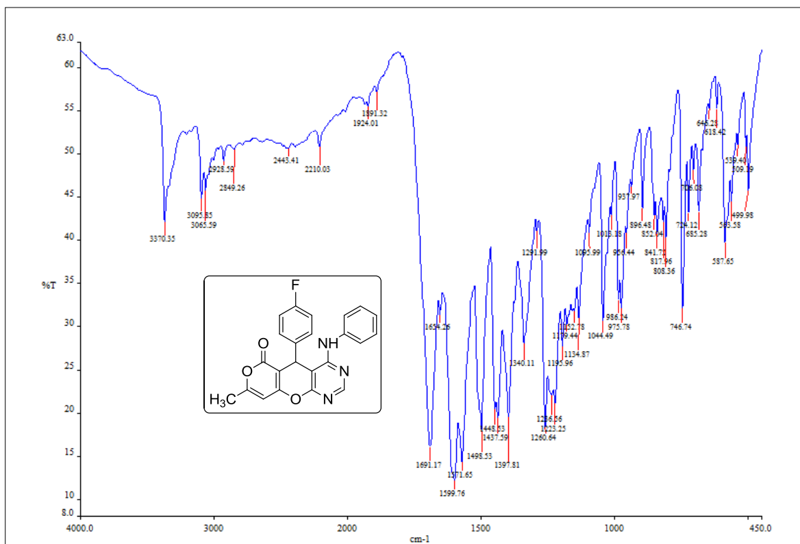
IR Spectrum of compound 4e
