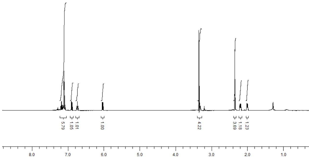
3h d.r. 96:4
