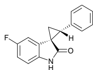
3m d.r.>99:1
