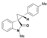
3h d.r. 96:4
