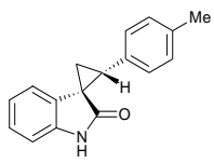
3p d.r. >99:1
