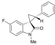
3c d.r. 96:4
