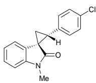
3g d.r.>99:1
