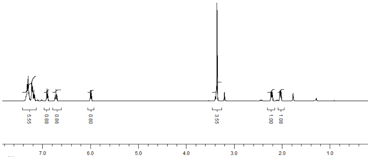
3a d.r. 93:7
