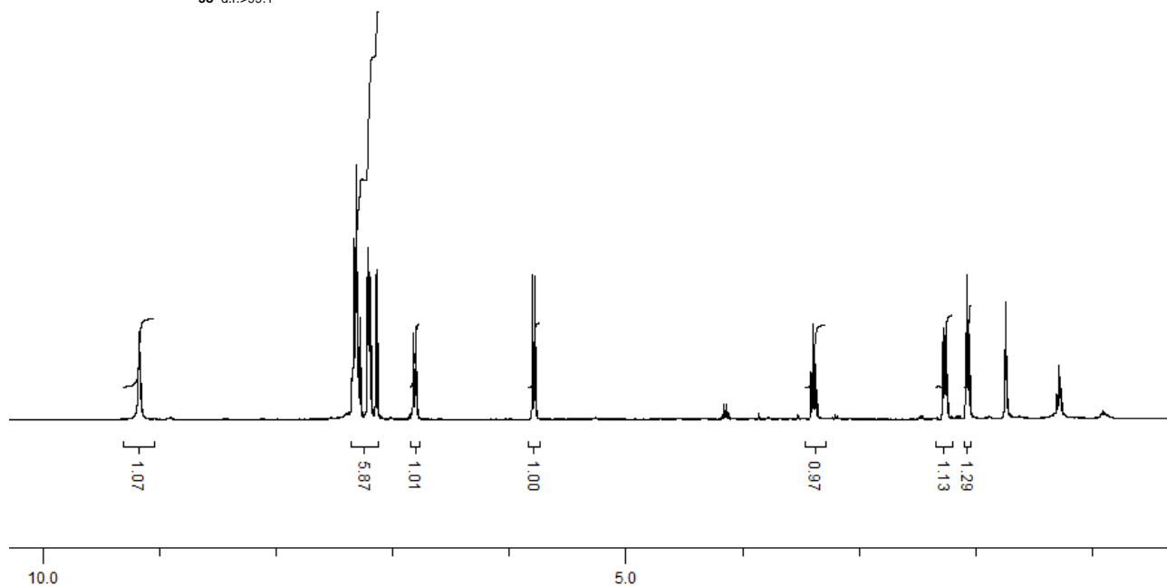
3o d.r.>99:1
