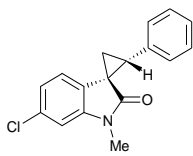
3d d.r.>99:1
