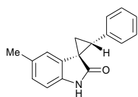
3n d.r. 98:2
