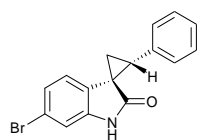
3o d.r.>99:1
