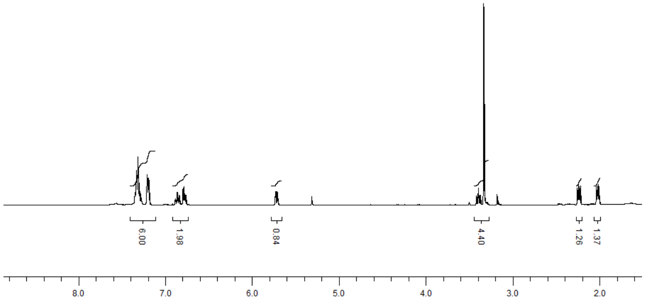
3c d.r. 96:4
