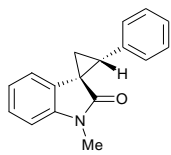
3a d.r. 93:7
