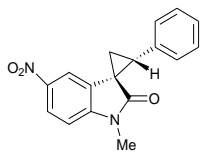
3f d.r. 98:2
