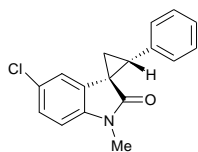
3b d.r. 94:6
