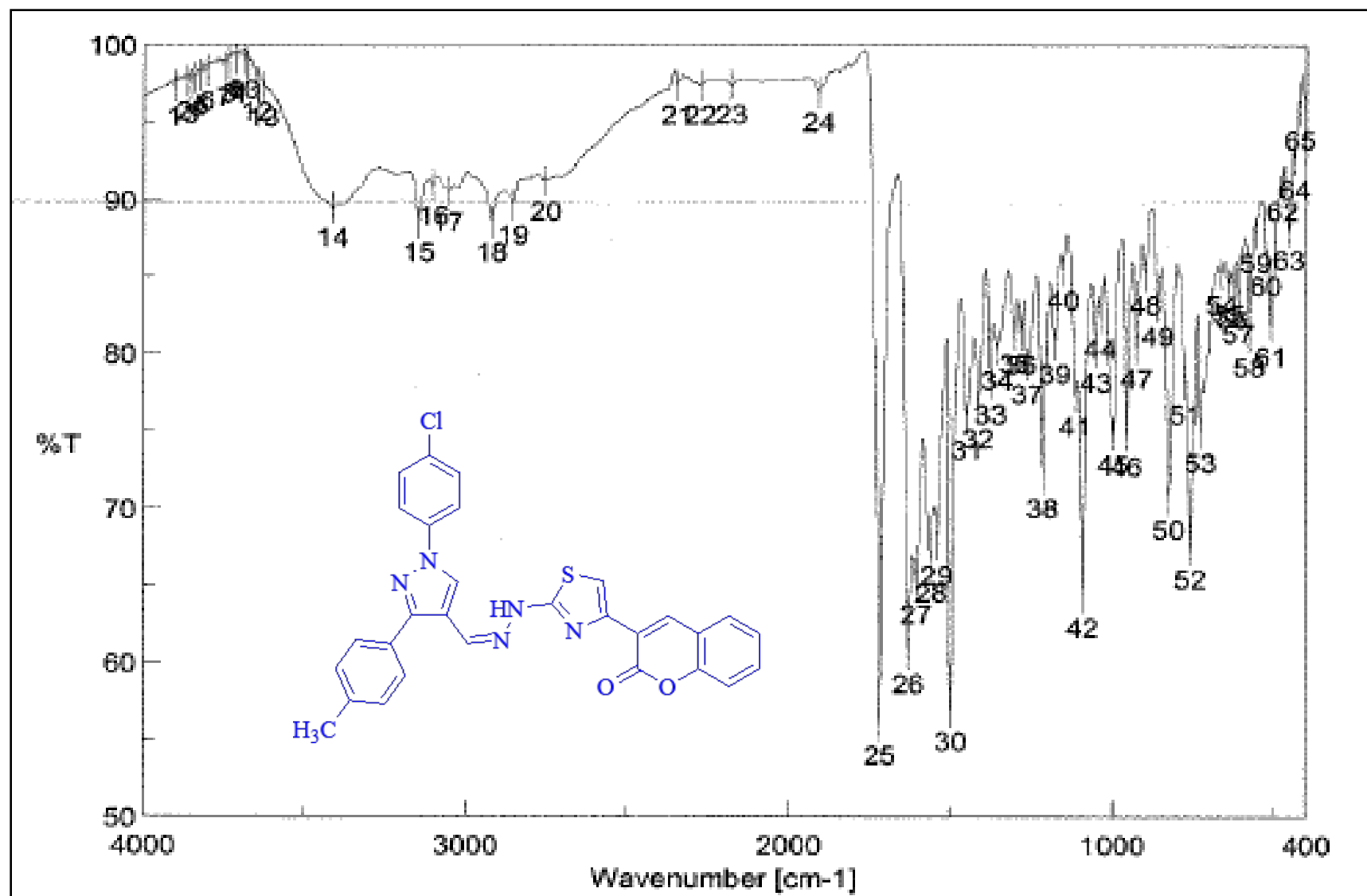
IR spectrum of 10d
