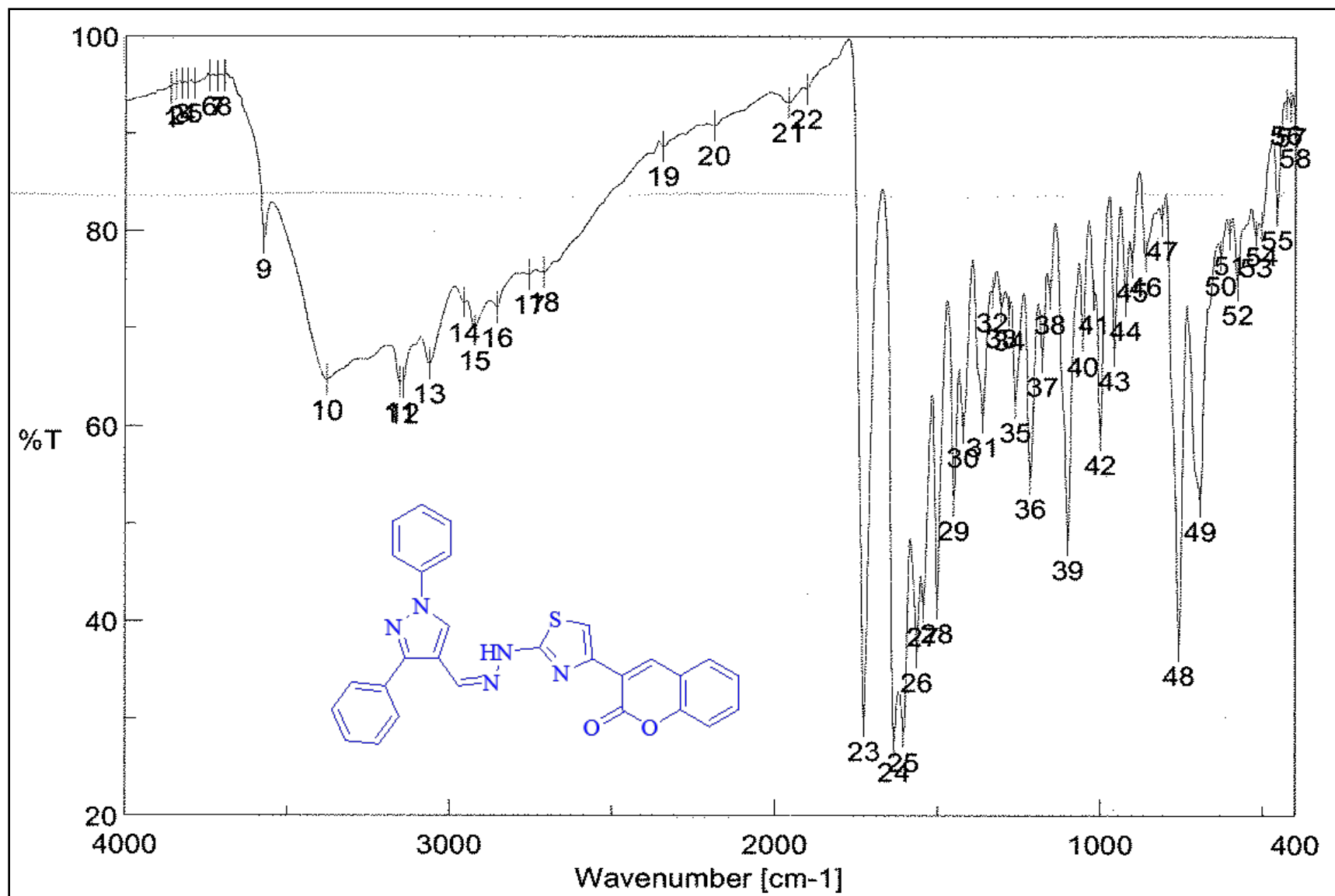
IR spectrum of 10a
