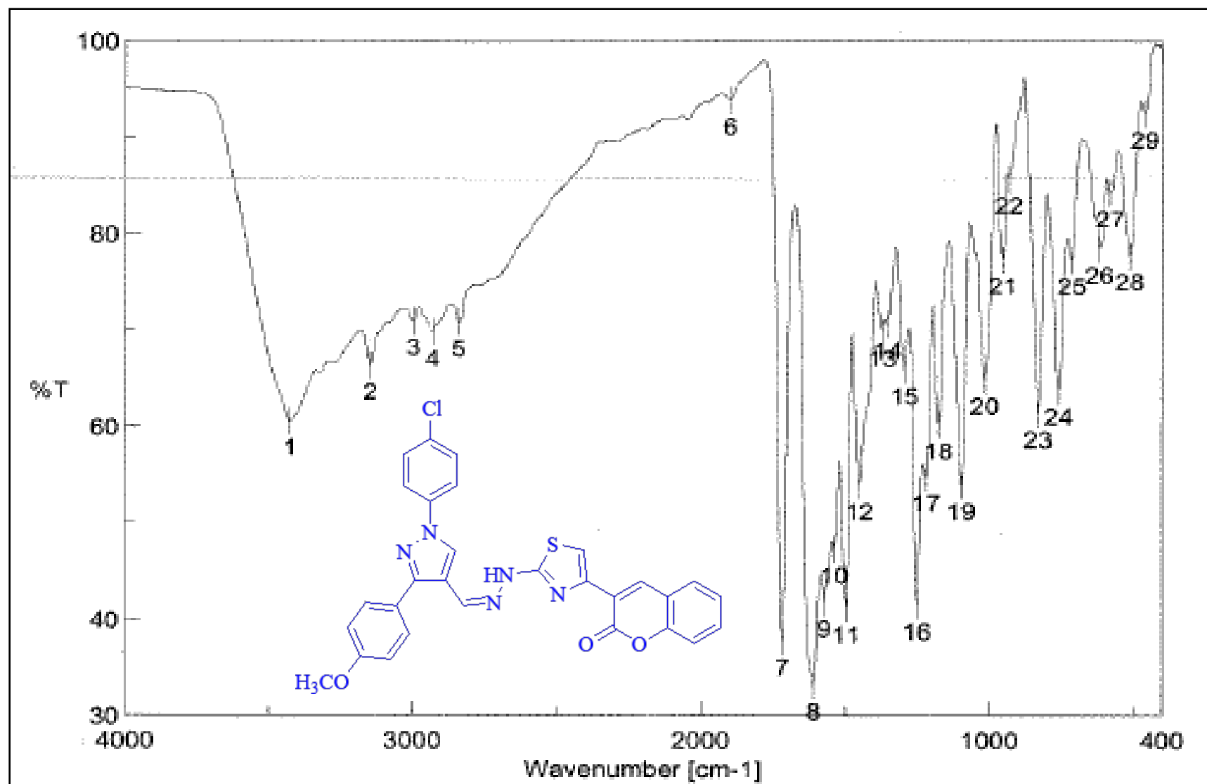
IR spectrum of 10f
