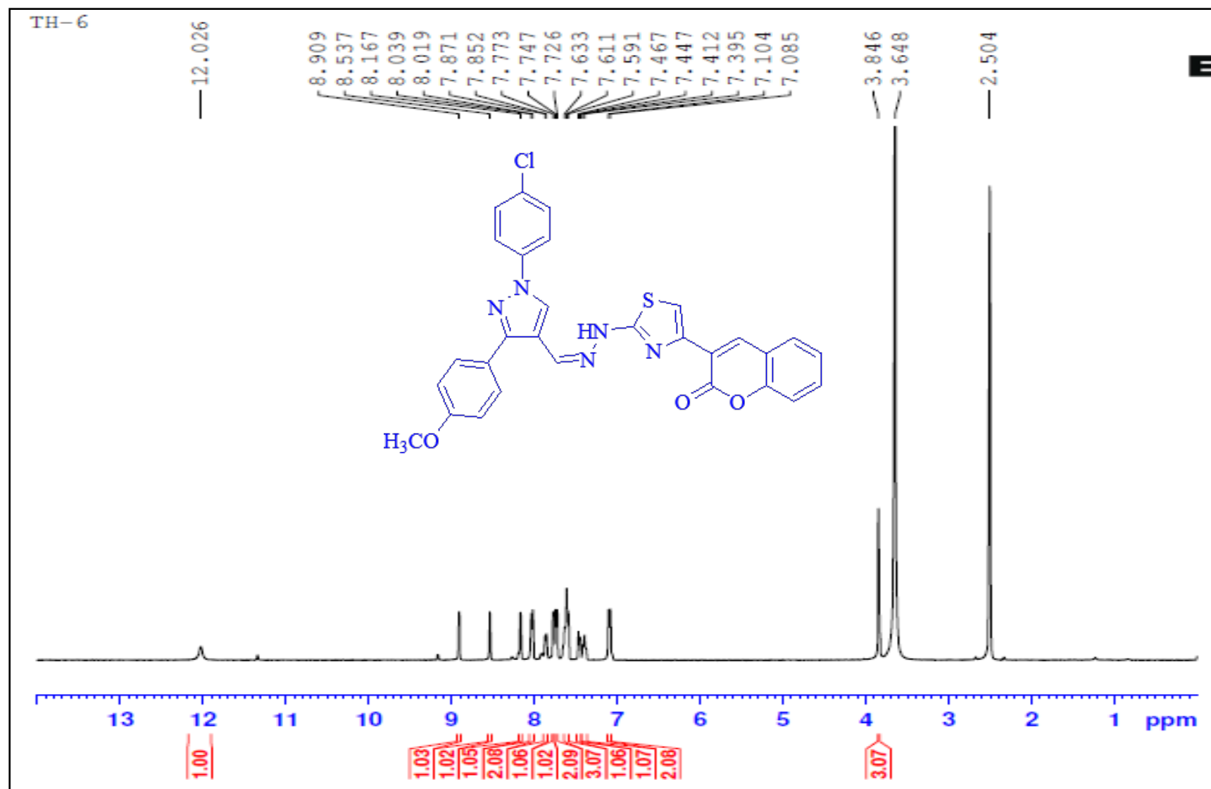
1 H NMR spectrum of 10f-DMSO-d 6 -400 MHz
