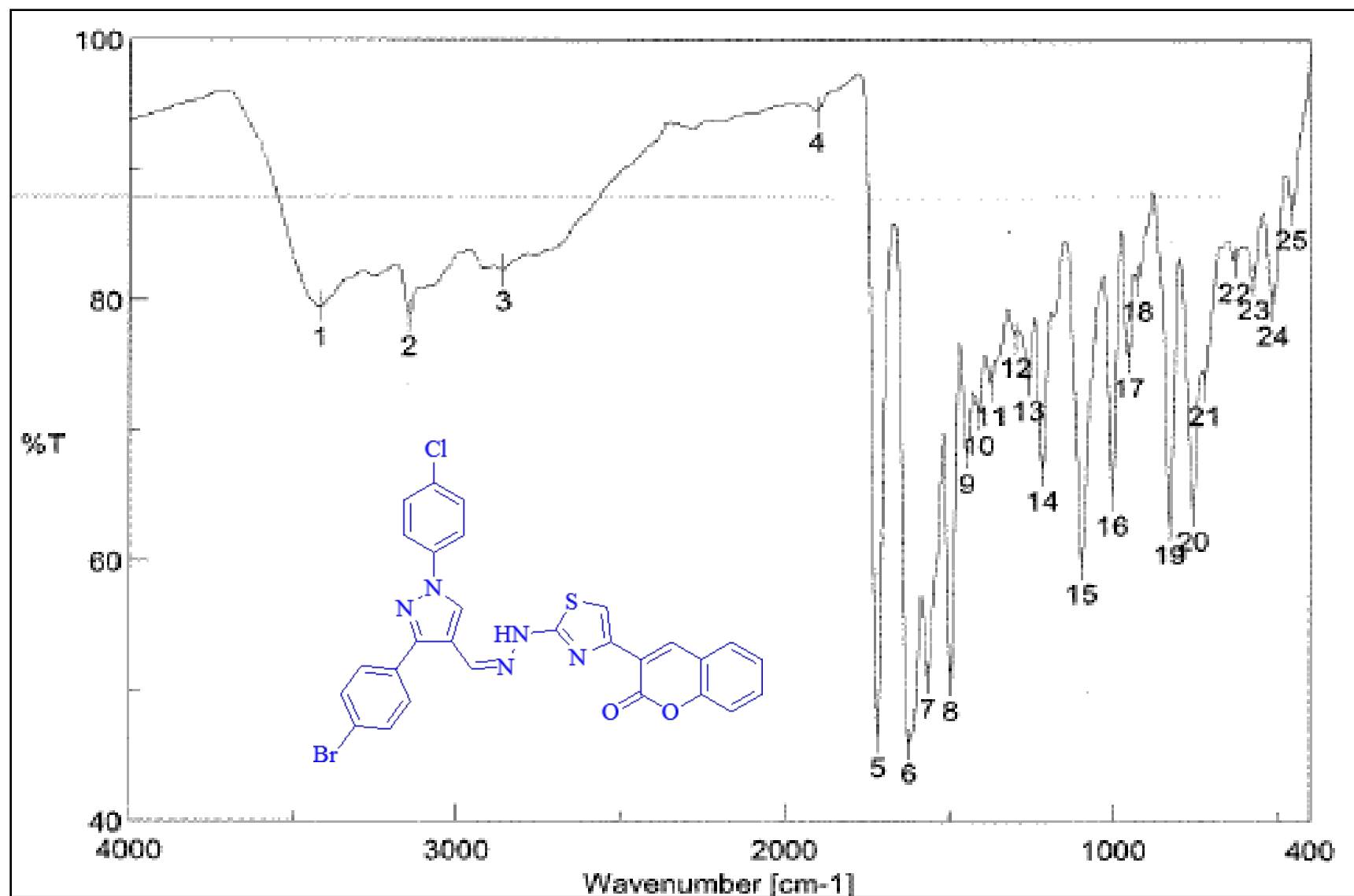
IR spectrum of 10j
