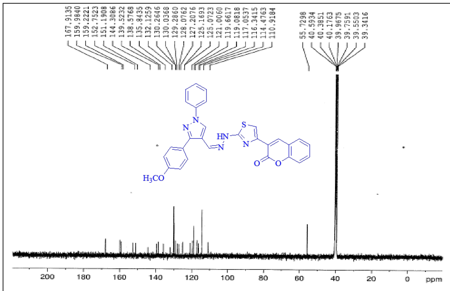
13 C NMR spectrum of 10e- DMSO-d 6 -100 MHz
