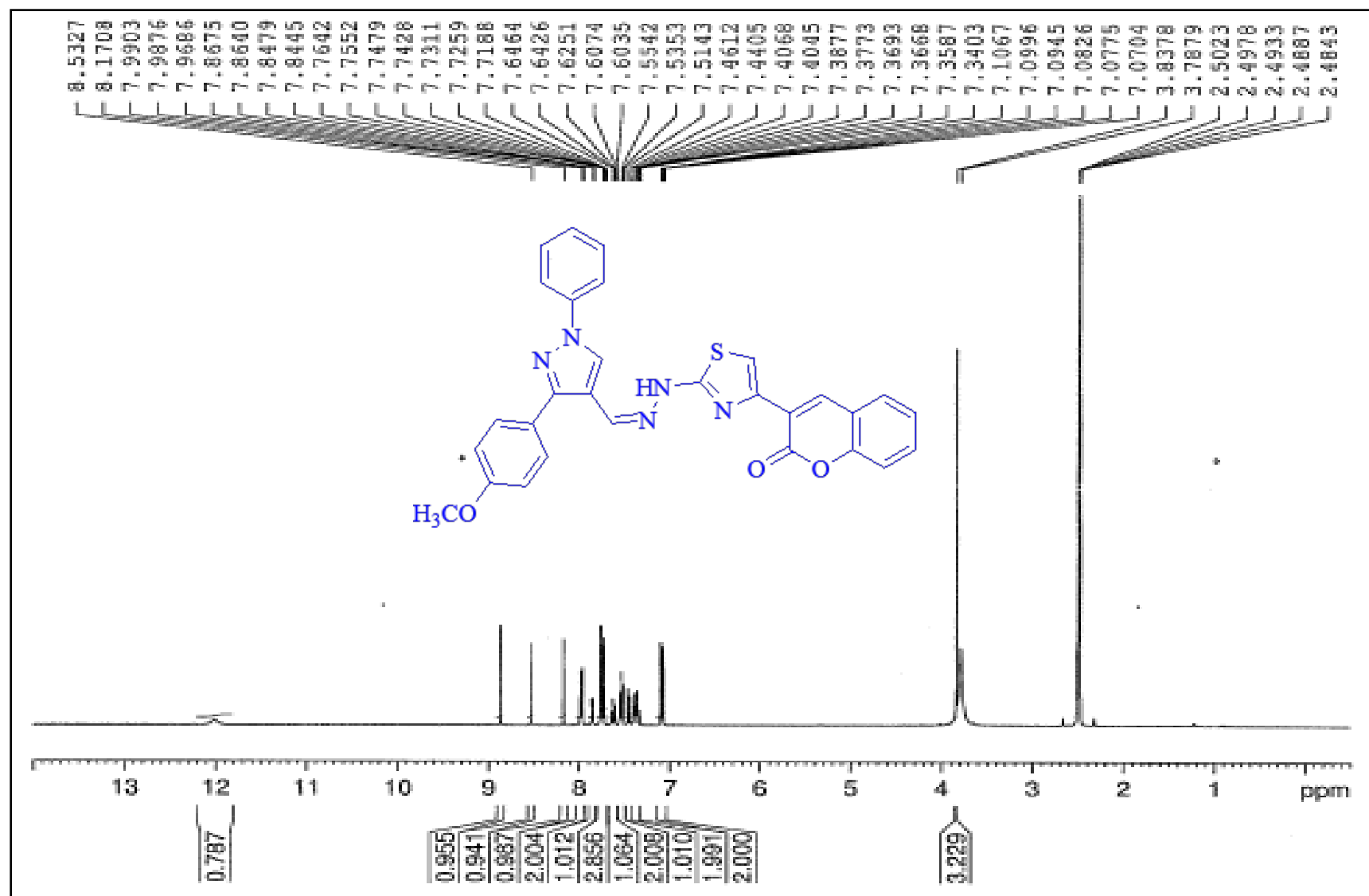
1 H NMR spectrum of 10e-DMSO-d 6 -400 MHz
