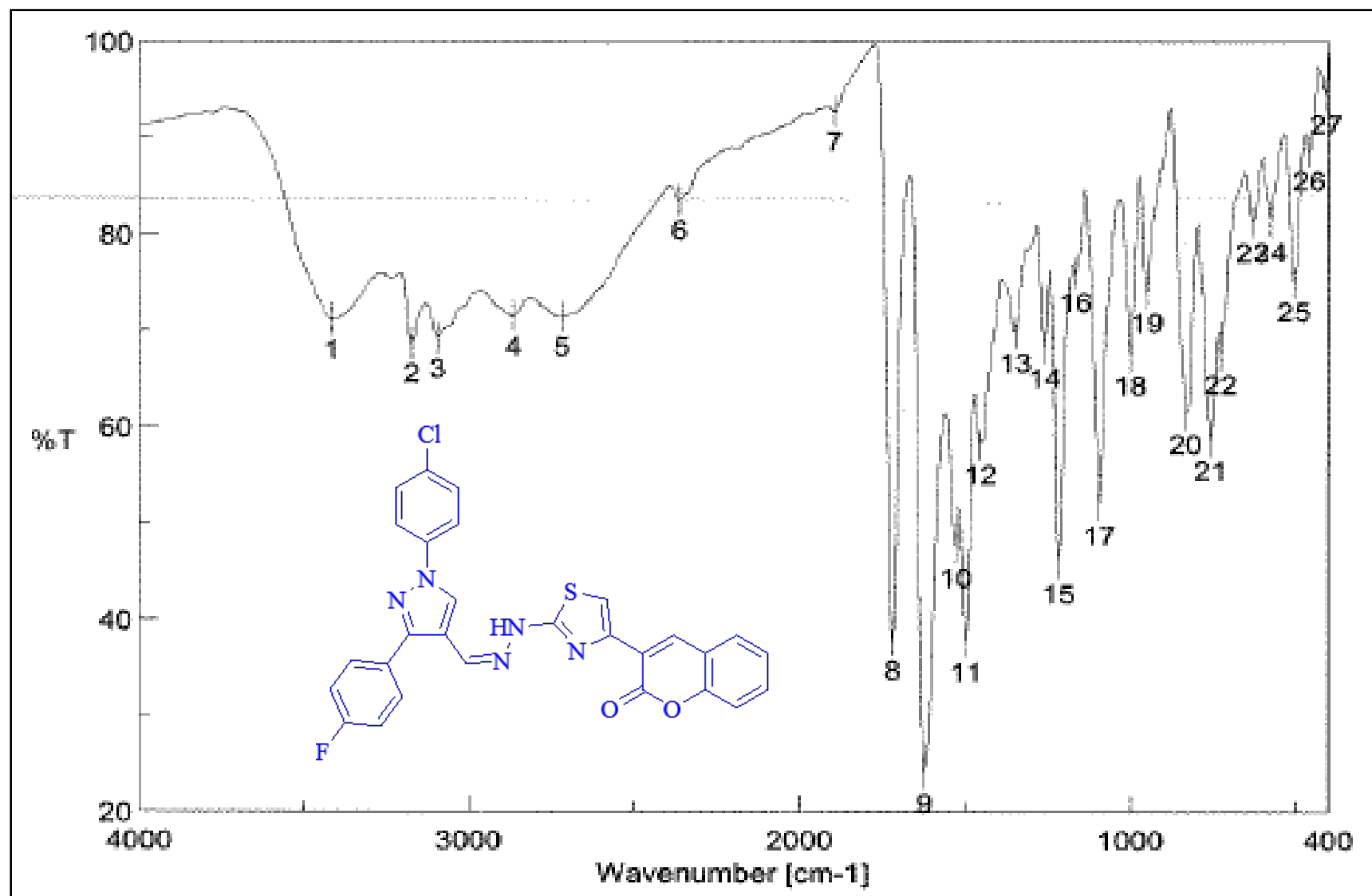
IR spectrum of 10l
