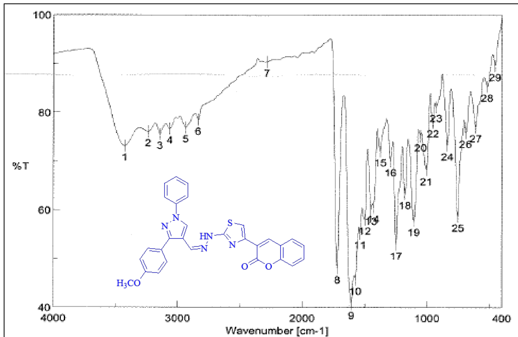
IR spectrum of 10e
