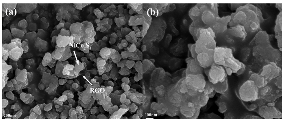
Fig. S1 FESEM images of NiCo 2 S 4 /RGO-3 hybrid.
