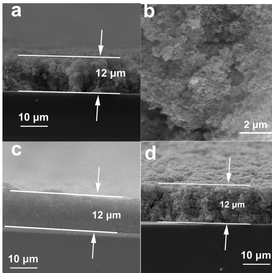
Figure S1. SEM images of the Hier-TiO 2 (a, b), Mes-TiO 2 (c), and Mac-TiO 2 (d)
