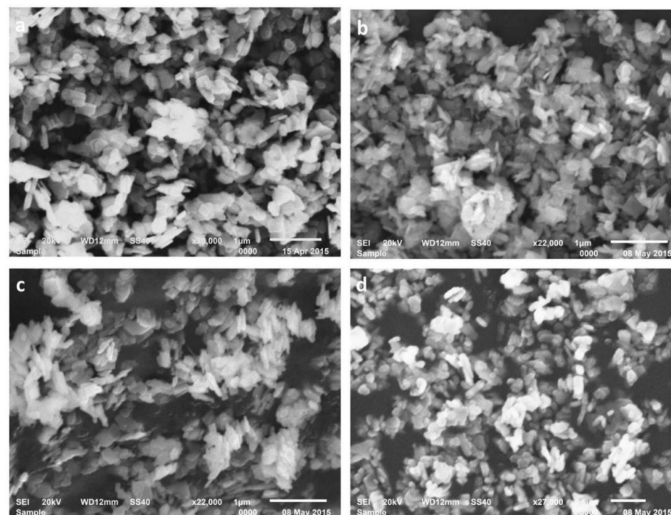
Fig. S1 SEM images of \text{Bi}_2\text{MoO}_6 (a), \text{Ag}/\text{Bi}_2\text{MoO}_6 (b), \text{Ag}_3\text{PO}_4/\text{Bi}_2\text{MoO}_6 (c) and \text{Ag}/\text{Ag}_3\text{PO}_4/\text{Bi}_2\text{MoO}_6 (d).
