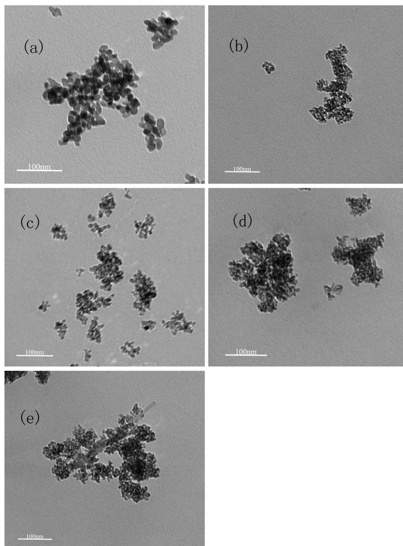
Fig. 2. TEM images of (a) ZrO_2 , (b) WO_x/ZrO_2 , (c) MoO_x/ZrO_2 , (d) SO_4^{2-}/WO_x-ZrO_2 and (e) SO_4^{2-}/MoO_x-ZrO_2
