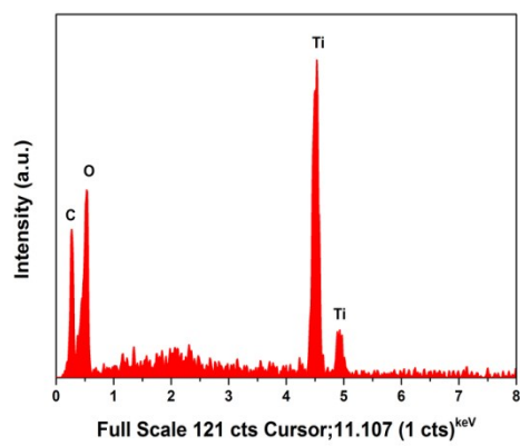
Fig. S2 EDS of 50wt% TiO 2 /CA composite
