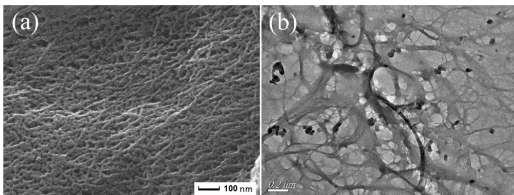
Fig. S1 (a) SEM and (b) TEM of CA
