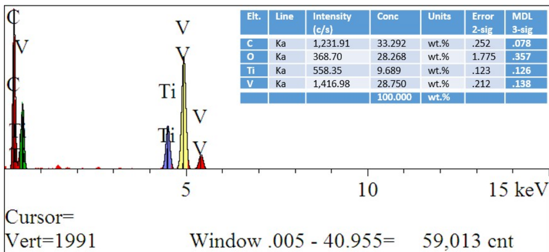
Figure S2 EDS of TiO_2 - V_2O_5 -CNT
