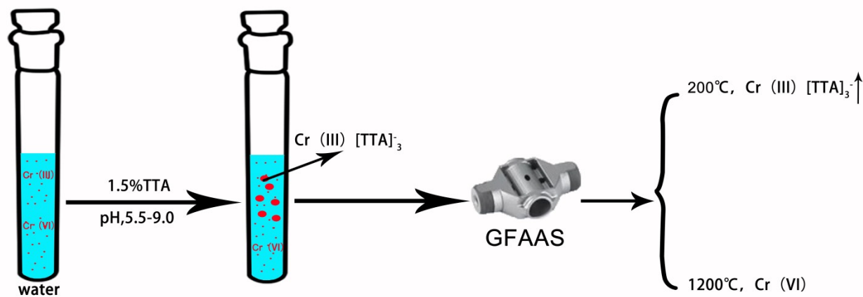
Fig. 1S. Procedure of in-situ thermal separation ETAAS.
