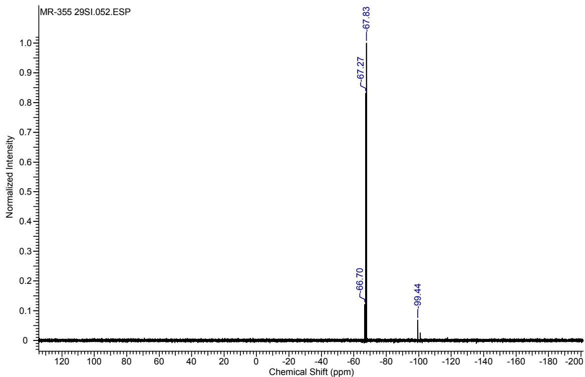
1-ethynyl-3,5,7,9,11,13,15-hepta(cyclopentyl)-pentacyclo[9.5.1.1 3,9 .1 5,15 .1 7,13 ]-octasiloxane (1B-c)
