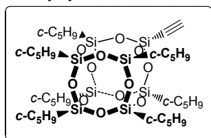
1-ethynyl-3,5,7,9,11,13,15-hepta(cyclopentyl)-pentacyclo[9.5.1.1 3,9 .1 5,15 .1 7,13 ]-octasiloxane (1B-c)
