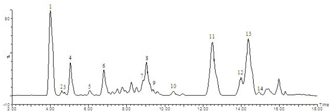
Fig.S1. UPLC chromatogram of SCE (1) schisandrin; (2) gomisin D; (3) gomisin J; (4) schisandrol B; (5) tigloylgomisin H; (6) angeloylgomisin H; (7) schisantherin A; (8) schisantherin B; (9) Schisanhenol; (10) gomisin E; (11) deoxyschizandrin; (12) gomisin N; (13) Schisandrin B; (14) Schisandrin C.
