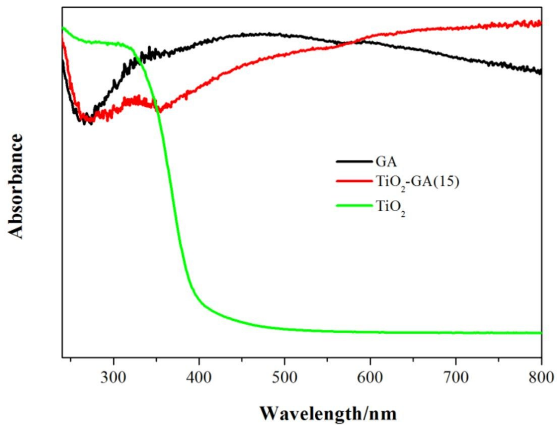
Fig. S1 DR UV-Vis spectra of pristine GA, TiO 2 , and TiO 2 -GA(15) composites.
