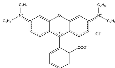
Fig. s2. The zwitter ion of Rhodamine B.
