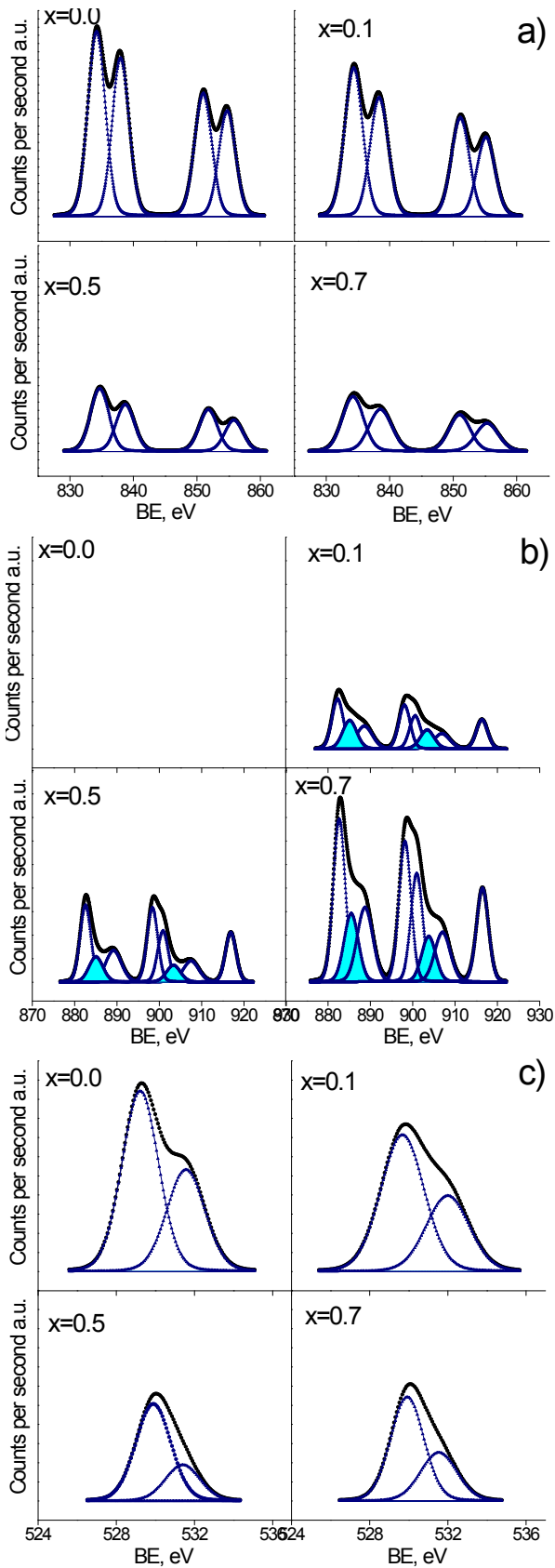
Appendix 2. a) La 3d; b) Ce 3d; c) O 1s
