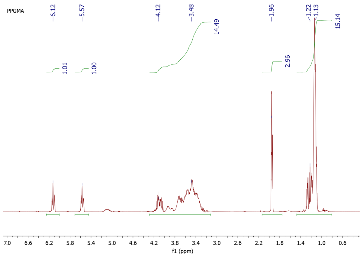
Fig. S1. 1 H NMR spectra of OPGMA macromonomer
