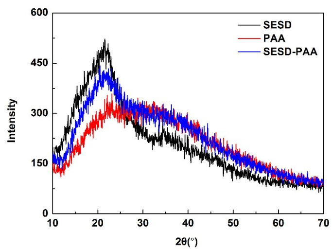
Fig. S1 XRD patterns of SEDS, PAA and SEDS-PAA.
