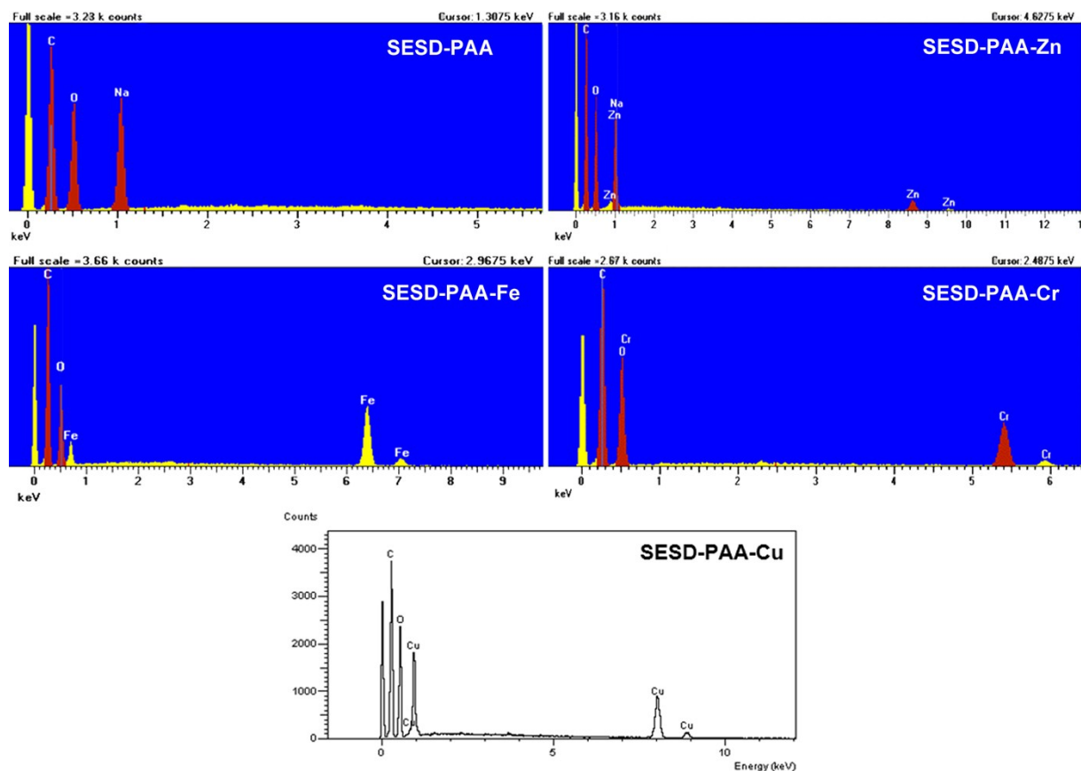
Fig. S2 EDX image of SEDS-PAA, SEDS-PAA-Zn, SEDS-PAA-Fe, SEDS-PAA-Cr and SEDS-PAA-Cu.
