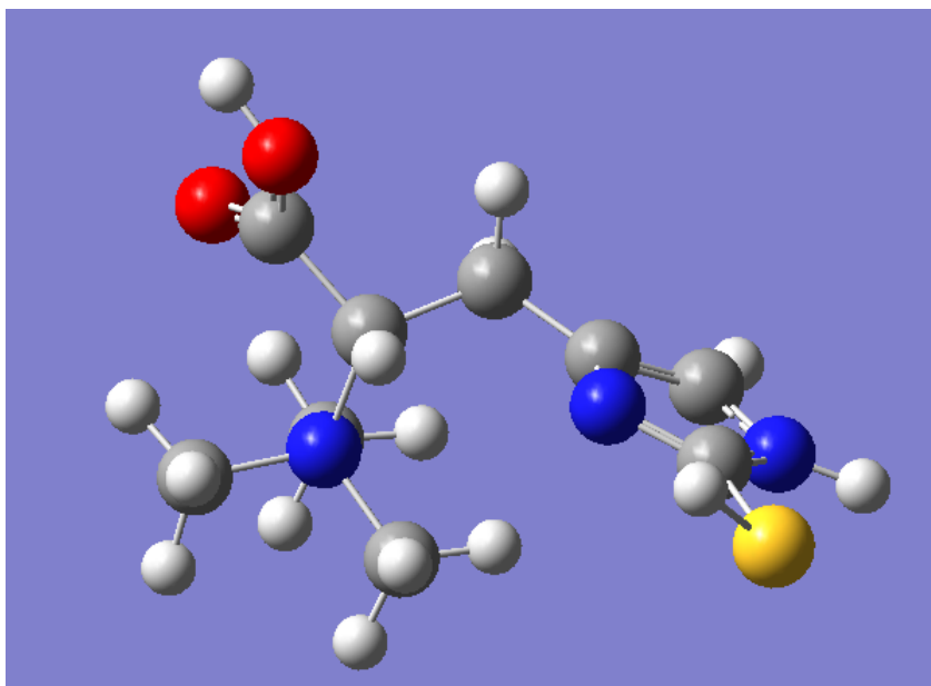
FIG. S3. Molecule
