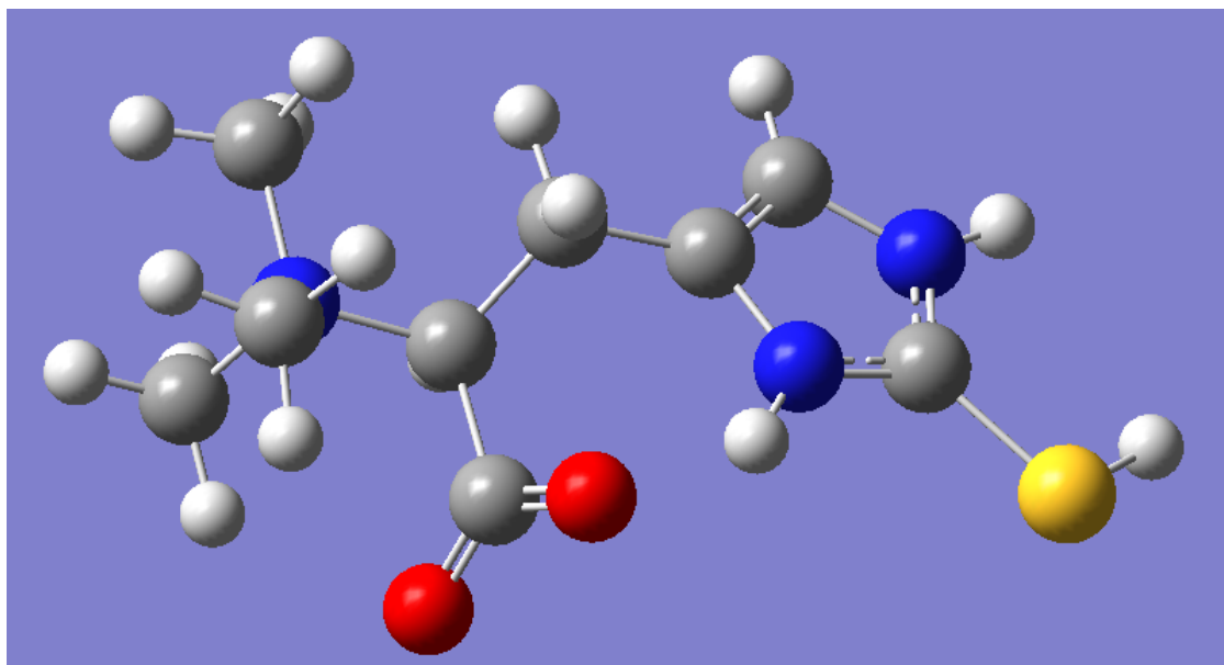
FIG. S4. Molecule
