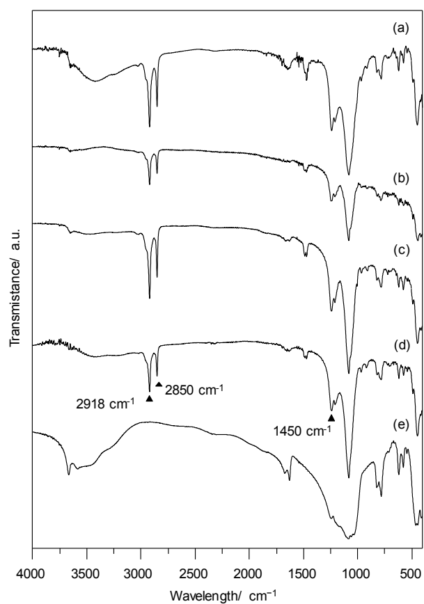
Figure S2. FT-IR spectra of CdSe(1)@CTA-magadiite (a), CdSe(0.5)@CTA-magadiite (b), CdSe(0.25)@CTA-magadiite (c), CTA-magadiite (d), magadiite (e).
