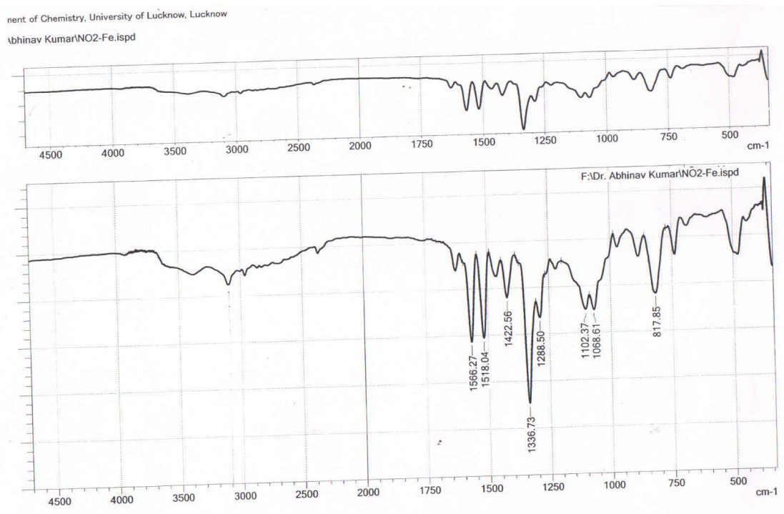
Fig. S6 IR spectrum of dye 2
