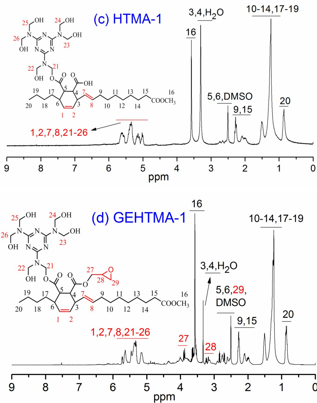
Fig. S1. ^1\text{H} NMR spectra of HHTT (a), TMA (b), HTMA-1 (c) and GEHTMA-1 (d)
