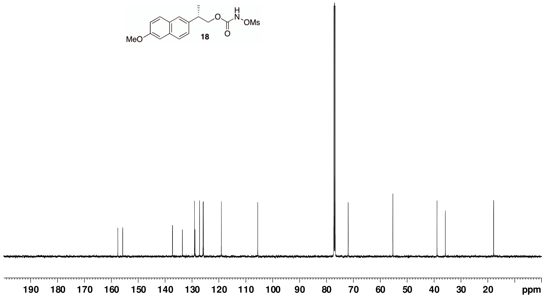
(S)-2-(6-Methoxynaphthalen-2-yl)propyl N-mesyloxycarbamate (18)
