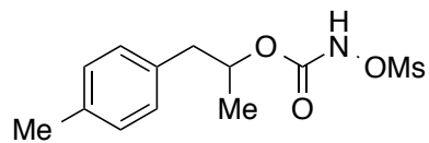
(±)-1-p-Tolylpropan-2-yl N-methylsulfonyloxycarbamate (S31)
