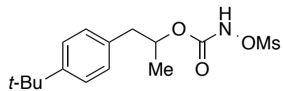
(±)-1-(4-(tert-Butyl)phenyl)propan-2-yl N-methylsulfonyloxycarbamate (S32)
