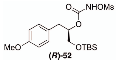
(R)-1-((tert-Butyldimethylsilyl)oxy)-3-(4-methoxyphenyl)propan-2-yl N-mesyloxycarbamate (52)
