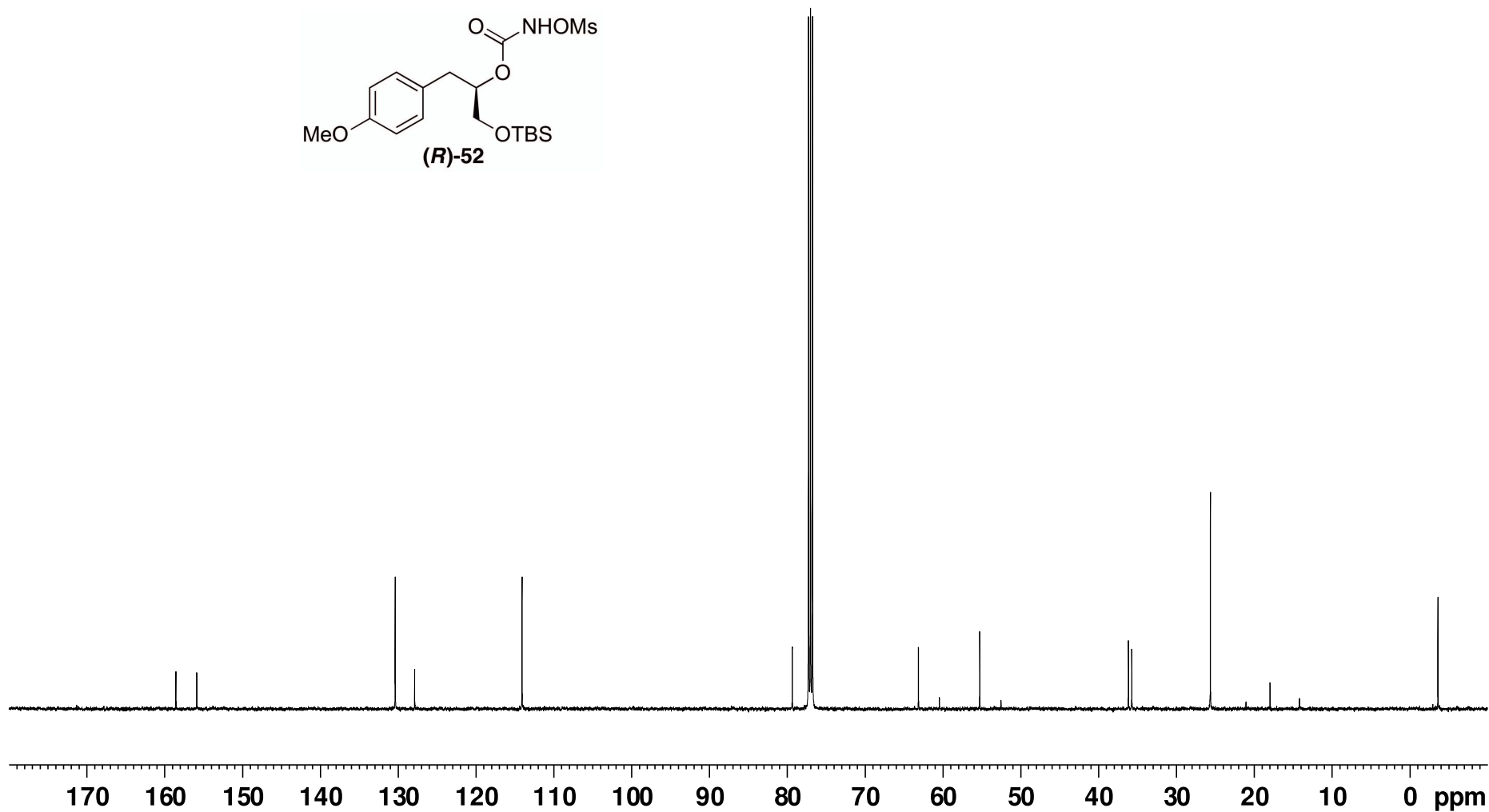
(R)-1-((tert-Butyldimethylsilyl)oxy)-3-(4-methoxyphenyl)propan-2-yl N-mesyloxycarbamate (52)
