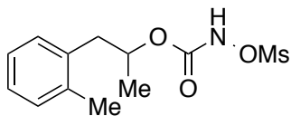
(±)-1-o-Tolylpropan-2-yl N-methylsulfonyloxycarbamate (S37)
