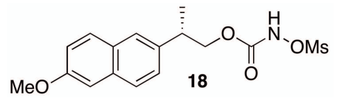
(S)-2-(6-Methoxynaphthalen-2-yl)propyl N-mesyloxycarbamate (18)
