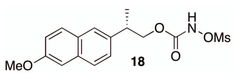
(S)-2-(6-Methoxynaphthalen-2-yl)propyl N-mesyloxycarbamate (18)
