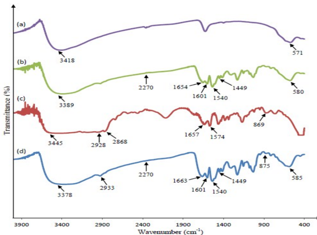
Fig. SI1 FT-IR spectra of (a) MNP, (b) MNP- \beta CD-TDI, (c) IL (BMIM-Cl) and (d) IL-MNP- \beta CD-TDI
