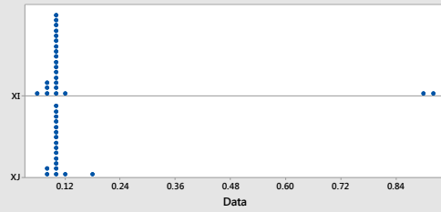
MnO
