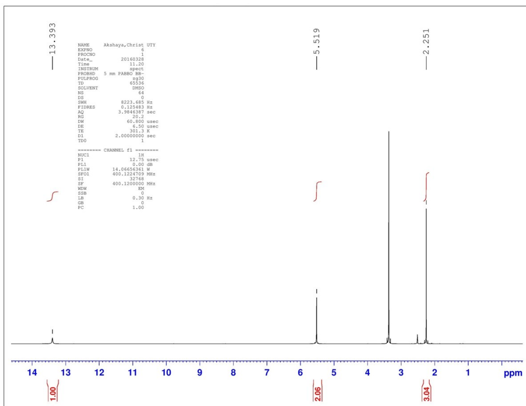
Fig. S1 1 H NMR spectrum of MMT.
