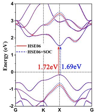
(d) a=3.148\text{\AA}
