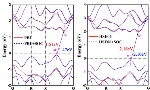
(d) a=3.148\text{Å}
