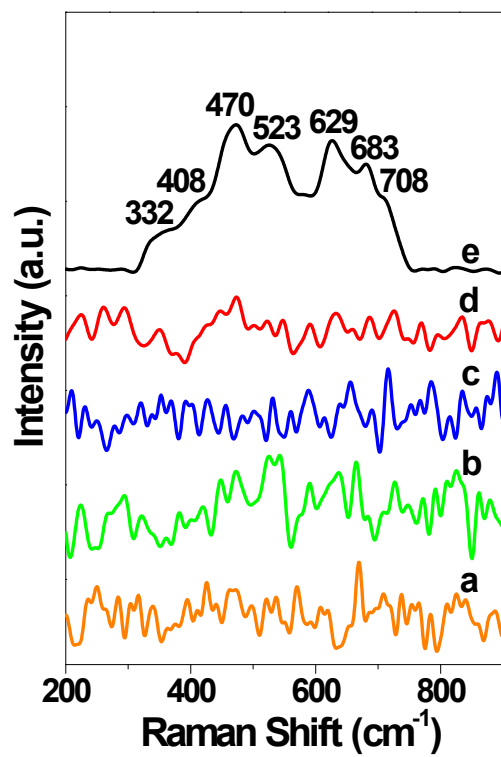
Fig. S1 Raman spectra of the (a) Ru/ASC(0.15), (b) Ru/ASC(0.39), (c) Ru/ASC(0.88), (d) Ru/ASC(2.35), and (e) Ru/AlOOH catalysts.
