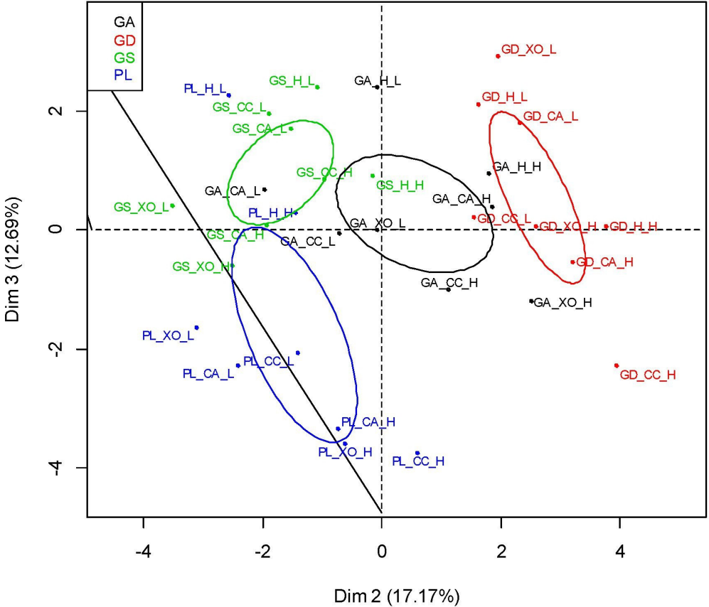
PCA_Fruits
