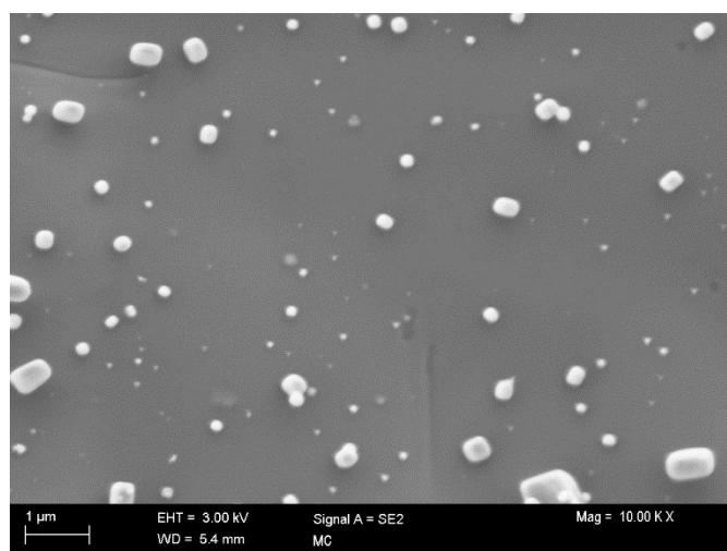
ESI Fig. 2. FESEM image of pure MC film
