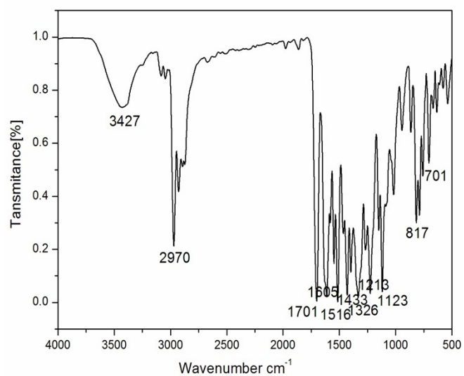
Fig. S2 IR of J1
