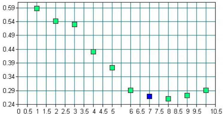
RMSECV vs Rang / HYCAGehalt+Verlust [mg] / Kreuzvalidierung
