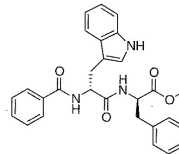
(2S,2'S)-6
