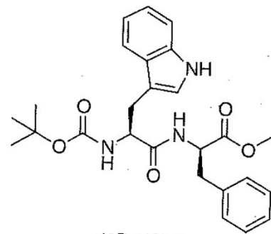
(2R,2'S)-8
