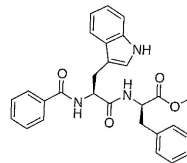
(2R,2'S)-6
