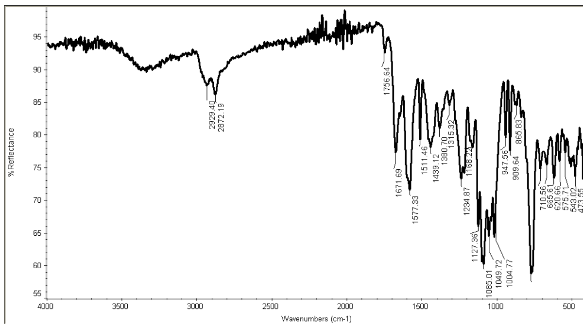
Fig. S1: IR spectrum of 6
