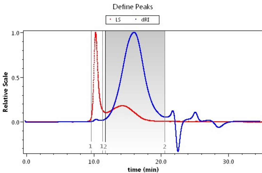
Fig. S4. GPC trace of PUE-0.
