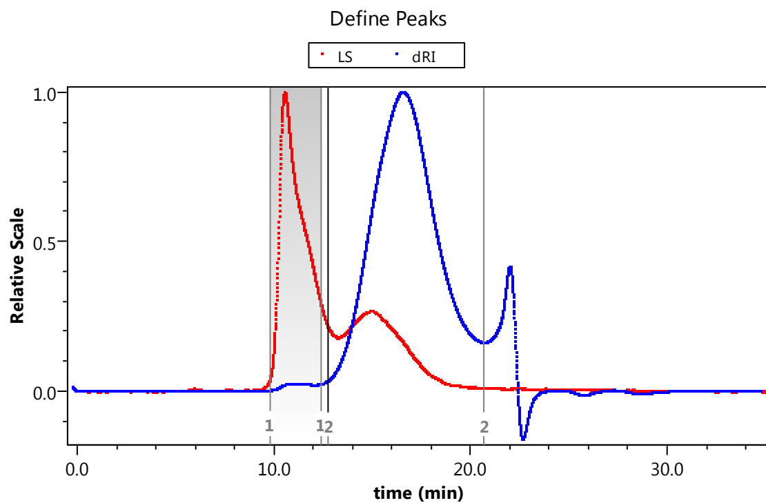
Fig. S3. GPC trace of PUE-C.
