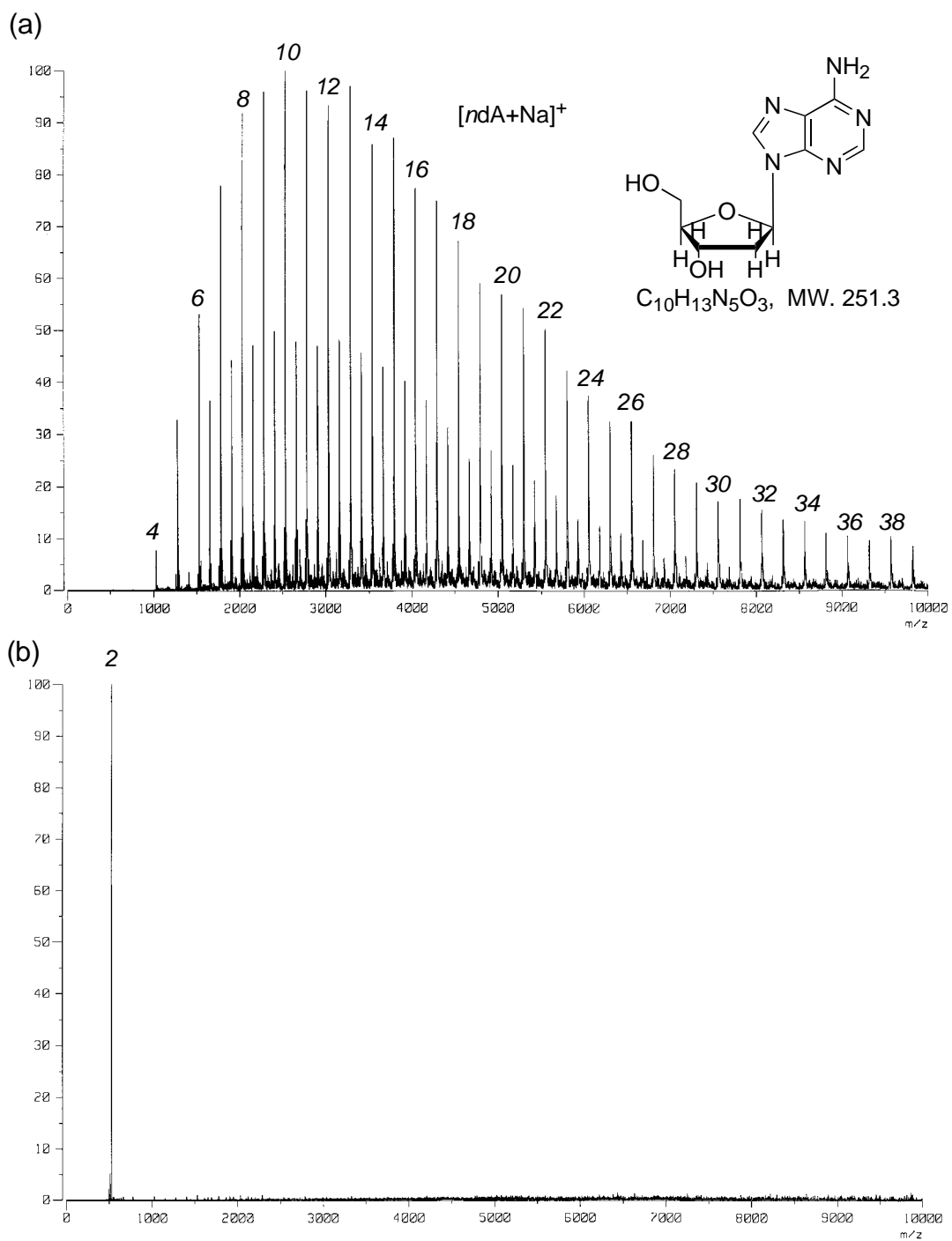
Figure S3 (a) CSI and (b) ESI-MS spectra of dA.
