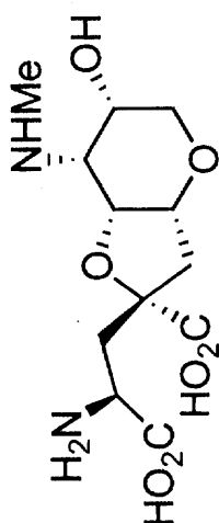
Dysiherbaine (Natural)
