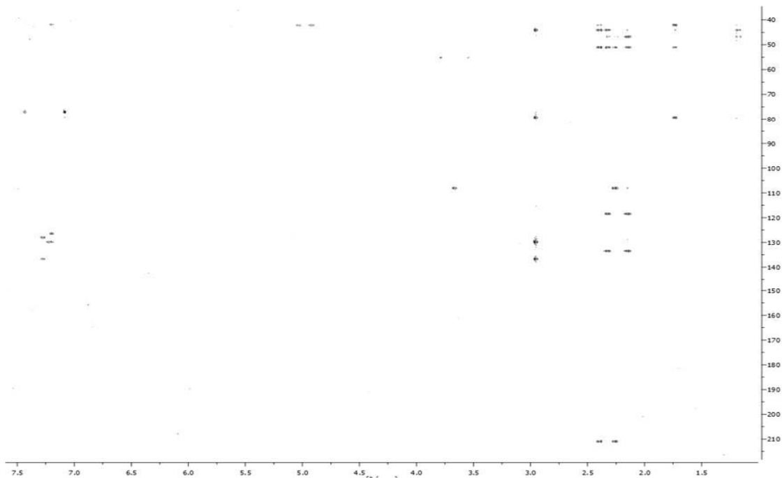
gHMBC-AD
