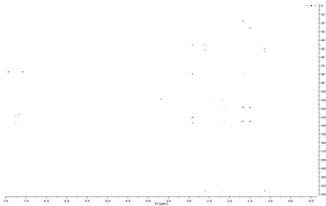
gHMBC-AD
