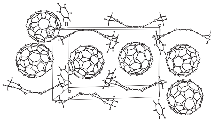
Figure S1. C_{70} \cdot ET \cdot C_6H_6 packing diagrams
